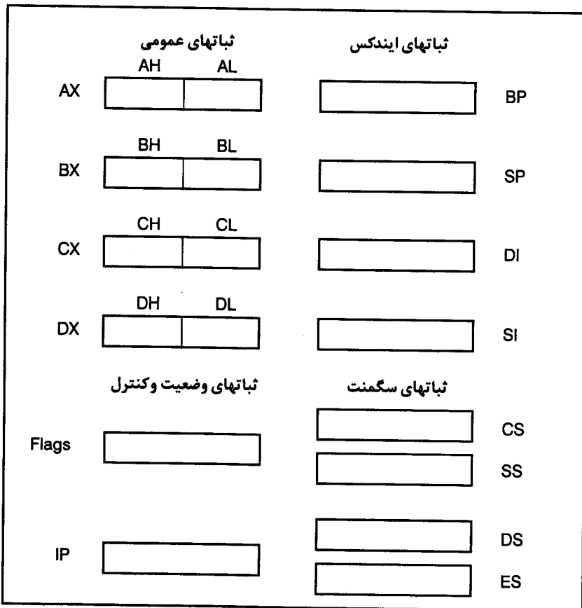
شکل ۲-۱۲ ثباتهای ۱۶ بیتی.
